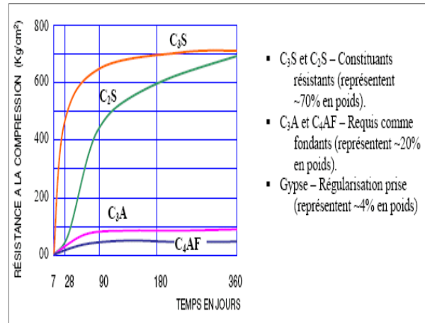
Figure. 3.13 (b): L'évolution des résistances des différents produits d'hydratation du ciment.
