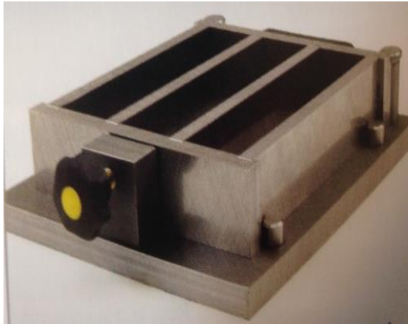
Figure. 3.13 (a): moule prismatique 4x4x16 pour essais de compression
