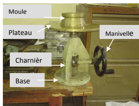
Figure 4.1 : Table à choc
