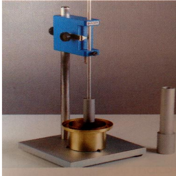
Figure 3.11 : Mesurer de la surface spécifique du ciment par l'appareil de Blaine
