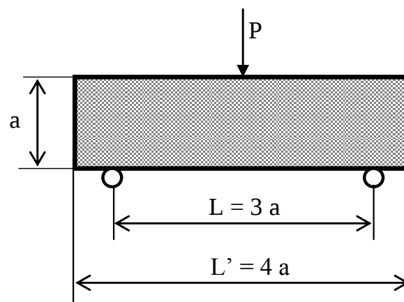
Figure 4.3 : Schéma de calcul de la flexion.
