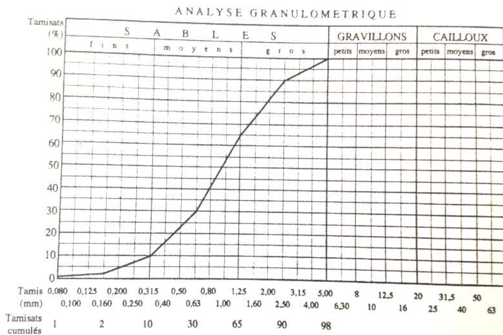
Figure 2.3 : Courbe granulométrique du sable étudié.
