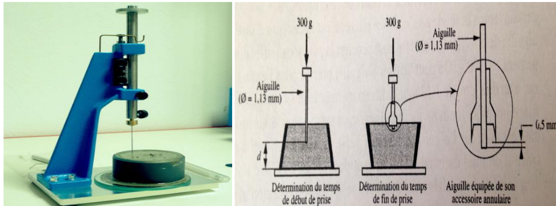
Figure 3.12 : Mesurer du temps de prise du ciment par l'appareil de Vicat
