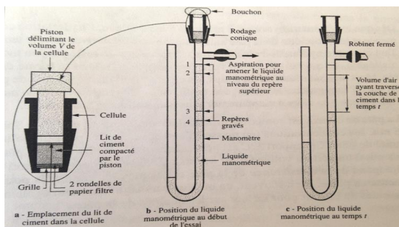
Figure 3.10 : Mesurer de la surface spécifique du ciment par l'appareil de Blaine.
