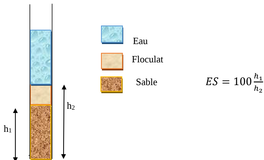
Figure 2.2 : Méthode de mesure de la propreté du sable.
